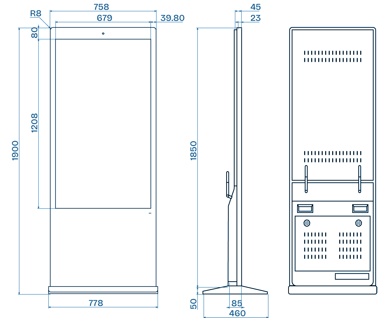
55" — 1900 X 758MM
